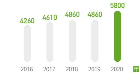
西电东送主网架通道能力 单位：万千瓦
